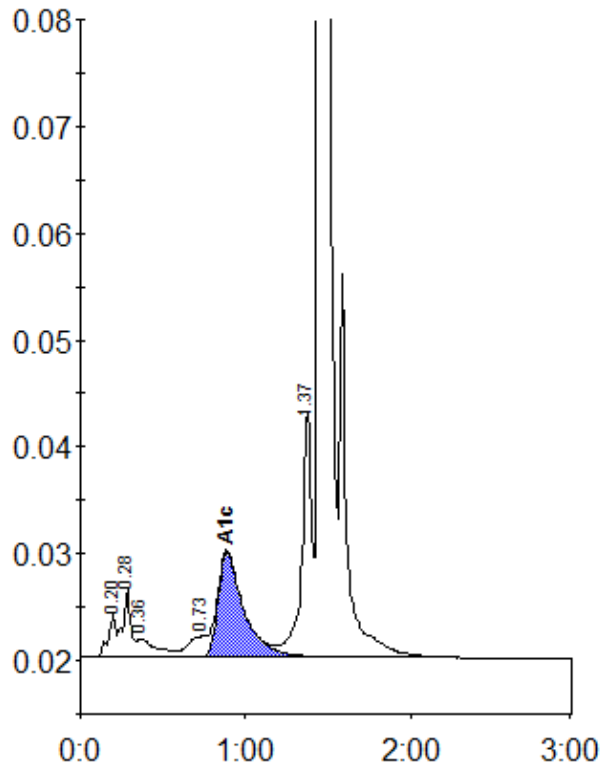
Peak table - ID: 10429699
